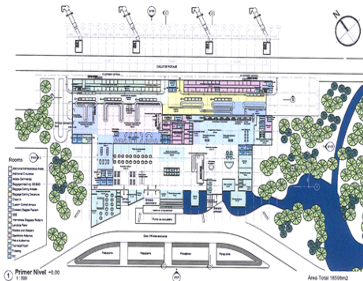
Ilustración 34 - Terminal diseño nivel 1 - fase 1
