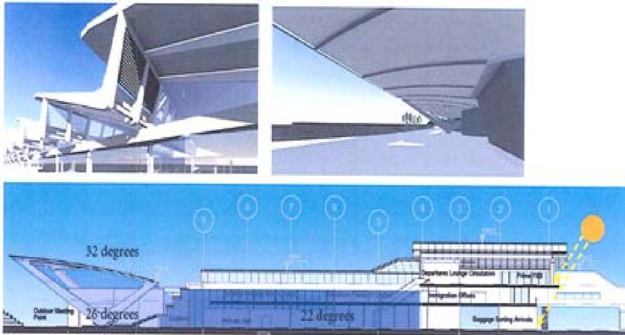
Ilustración 29 - Iluminación solar
