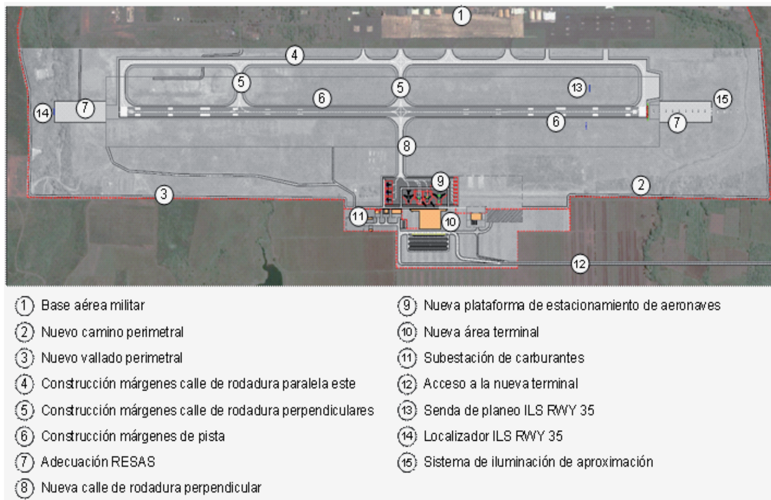
Figura 10: Esquema del proyecto de aeródromo
