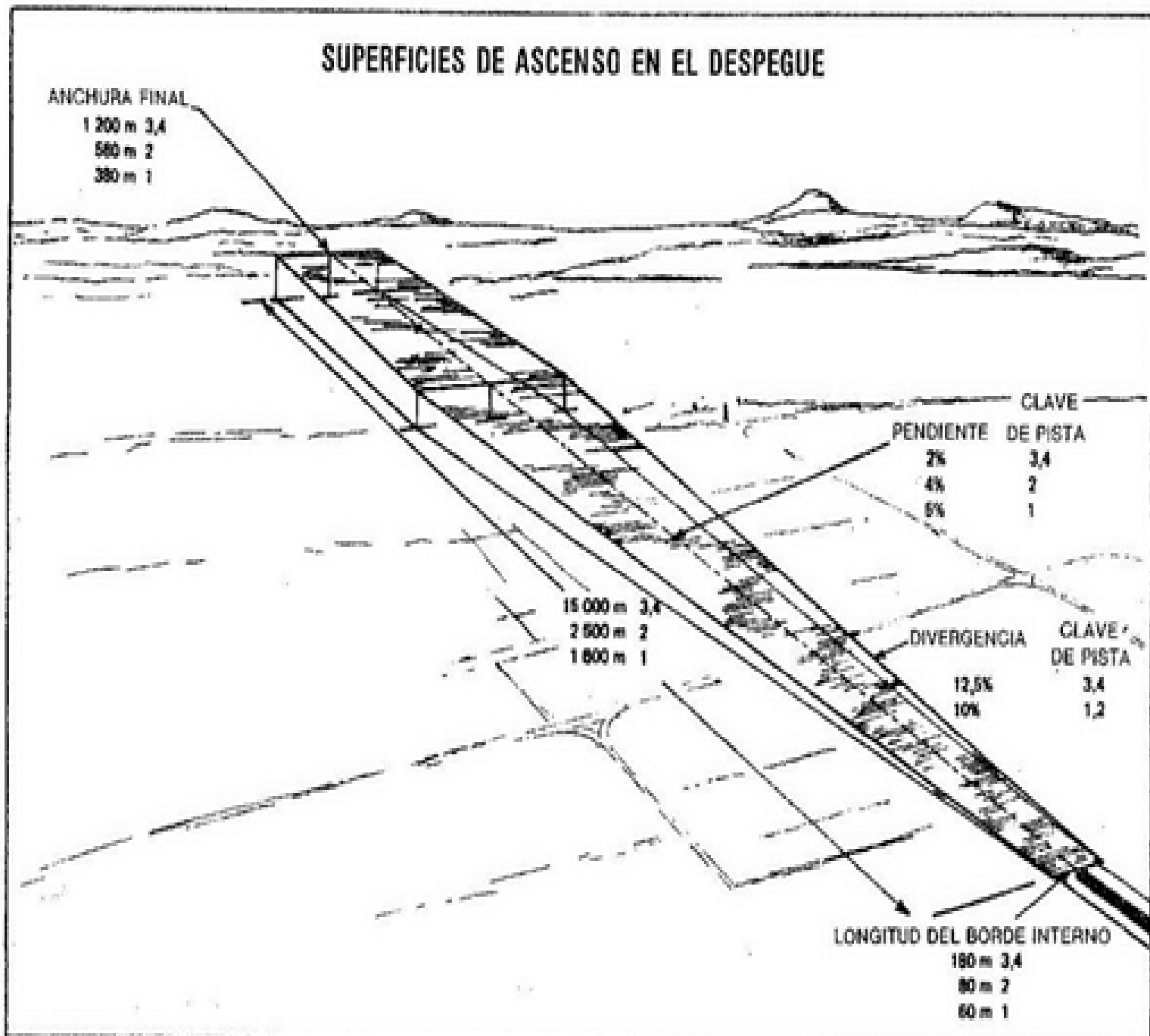
Figura 9. Superficie de Ascenso en el Despegue
